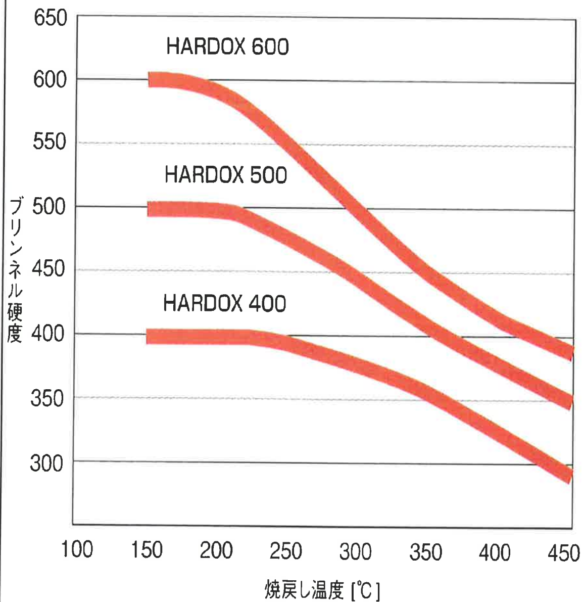
図2 表面硬度と焼戻し温度との関係
